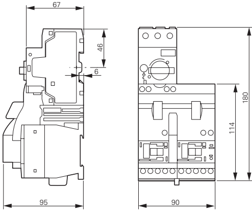
MSC-R-...-M7[...12]BBA...
