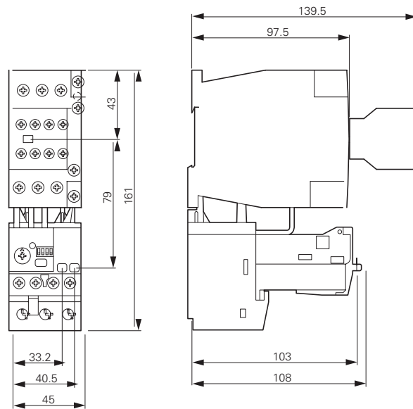
ZEB32
