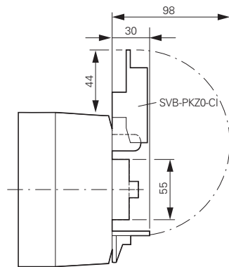
CI-PKZ0...M + SVB-PKZ0-CI
