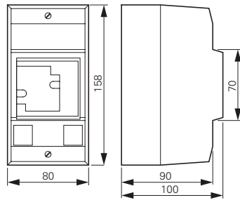
CI-PKZ0-M
