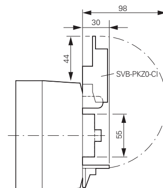
CI-K2-PKZ0-G(R)(V) + SVB-PKZ0-CI
