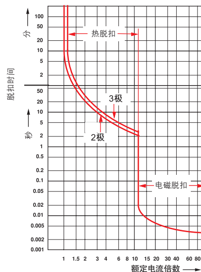
MSx脱扣曲线图
