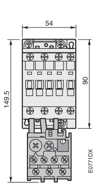
AX32, AX40 +TA25DU-M热过载继电器
