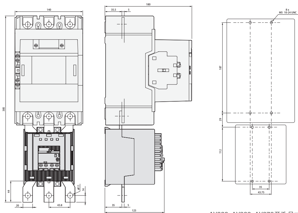
AX260, AX300, AX370 +EF370电子过载继电器
