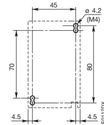
AX32, AX40开孔尺寸图
