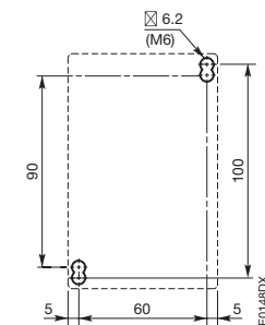
AX50, AX65, AX80开孔尺寸图
