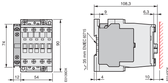
AX32, AX40 +CAL5X侧装2极辅助触点模块
